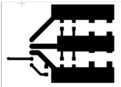
Fig. 2a. Layer 1 conductor.
