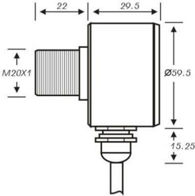
图 5-1b 外型尺寸
