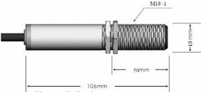
图 5-1a 外型尺寸
