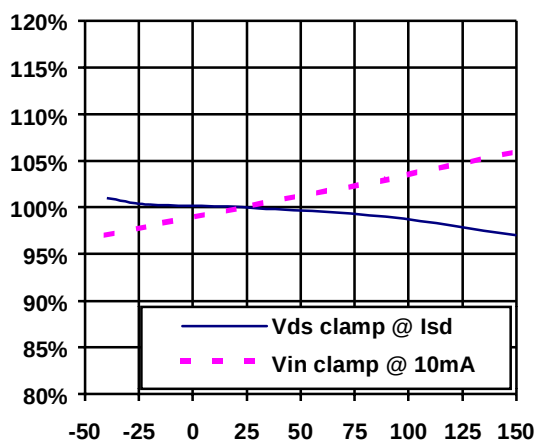
Figure 19 - Vin clamp1 & Vin clamp2 (%) Vs T J (°C)
