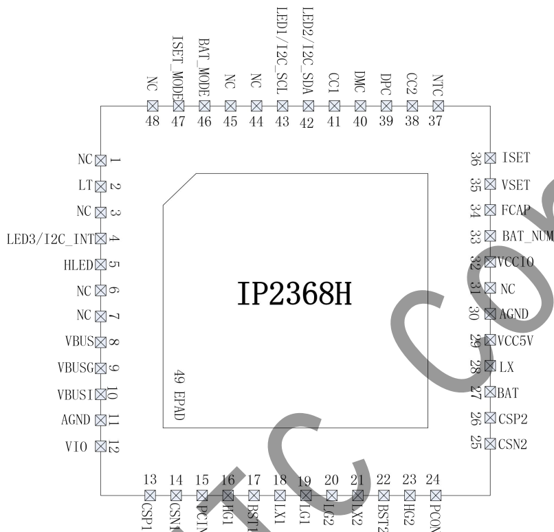
图 2 IP2368H 引脚图
