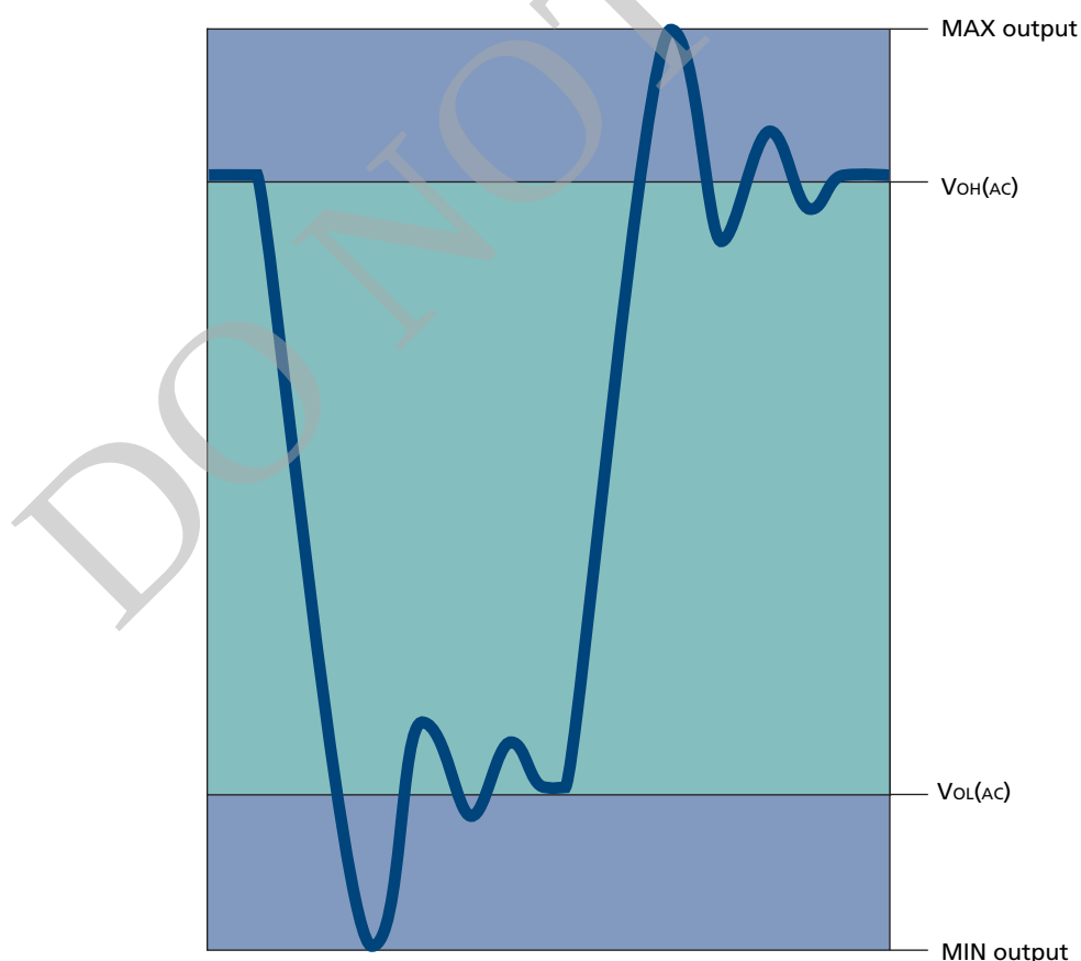
Figure 28: DQ Output Signal
