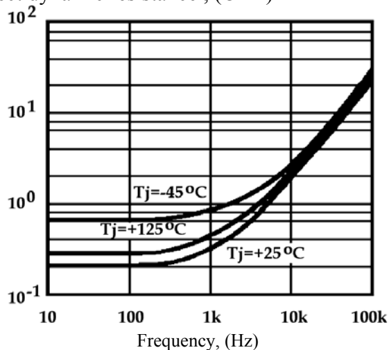
Figure 7 – Dynamic resistance versus frequency Зависимость динамического сопротивления от частоты
