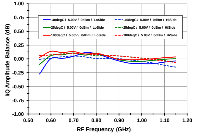
I/Q Amplitude Error vs. T CASE
