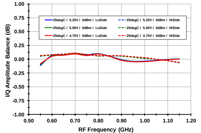
I/Q Amplitude Error vs. V CC
