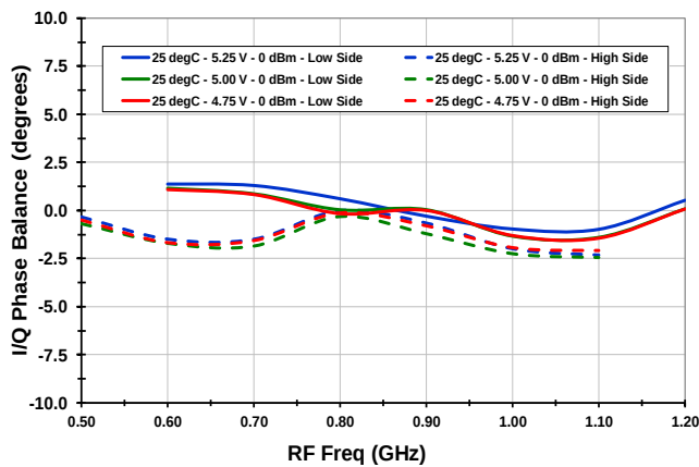
I/Q Phase Error vs. V CC
