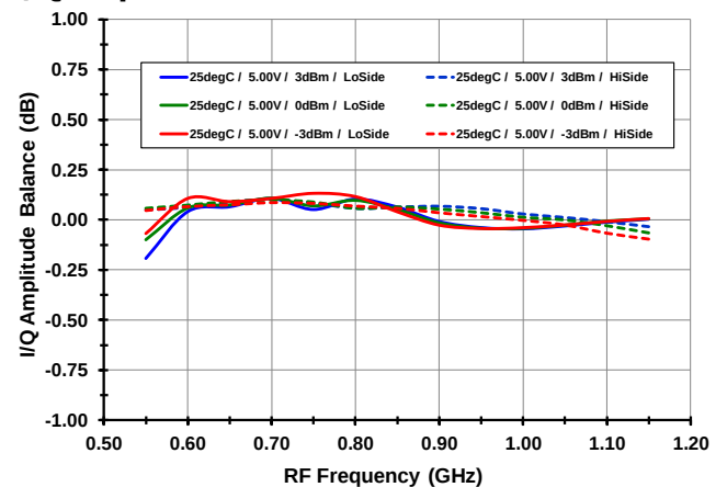
I/Q Amplitude Error vs. LO level
