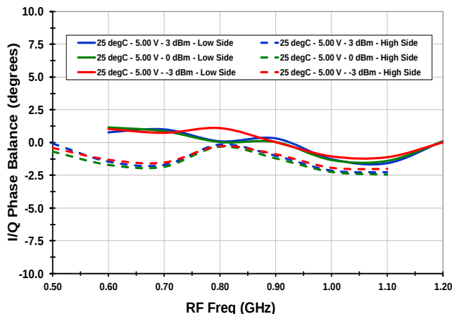
I/Q Phase Error vs. LO level
