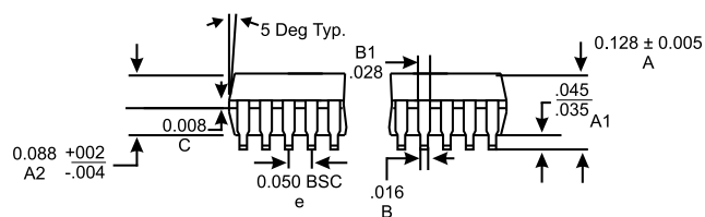
SOJ Package
