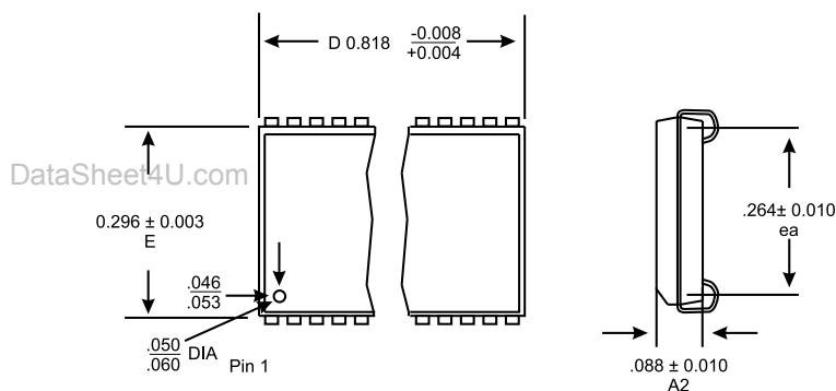
SOIC Package
