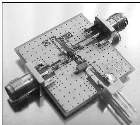
ICL2001-23 EVAL
