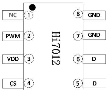
图 5.1 Hi7012 管脚图
