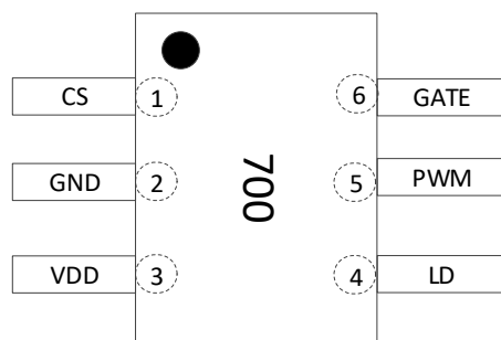
图 5-1 Hi7000D 管脚图
