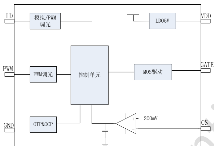
图 7-1 结构框图
