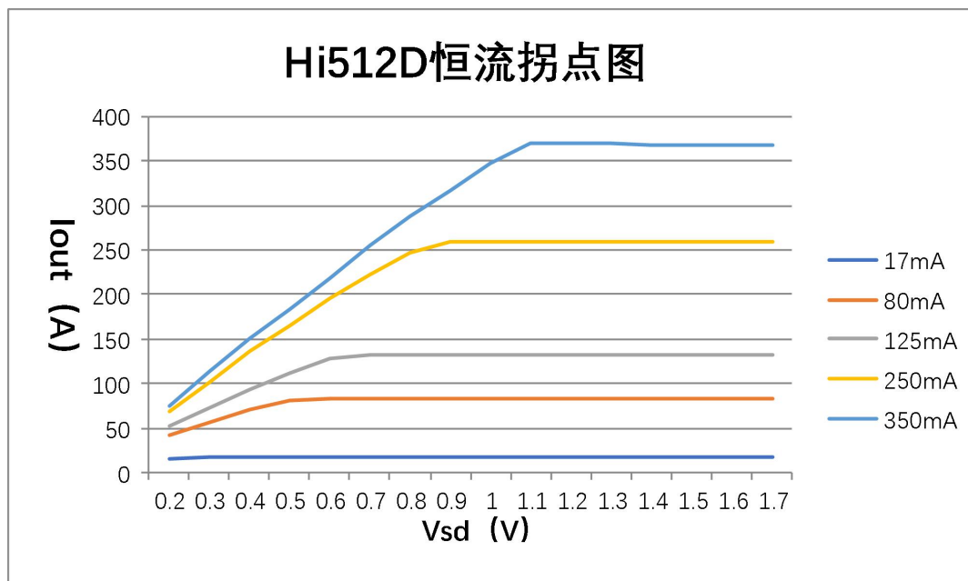
图 10.1 恒流拐点
