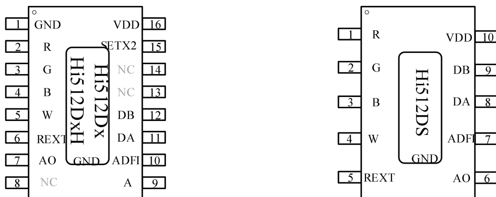
图 5.1 管脚图
