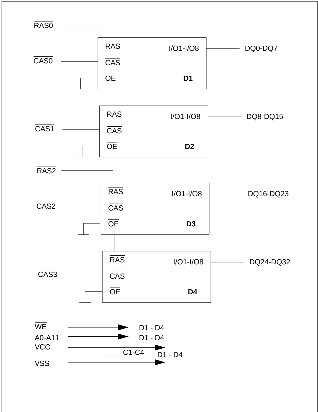
Block Diagramm
