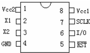
图 1 HYM1302 引脚图
