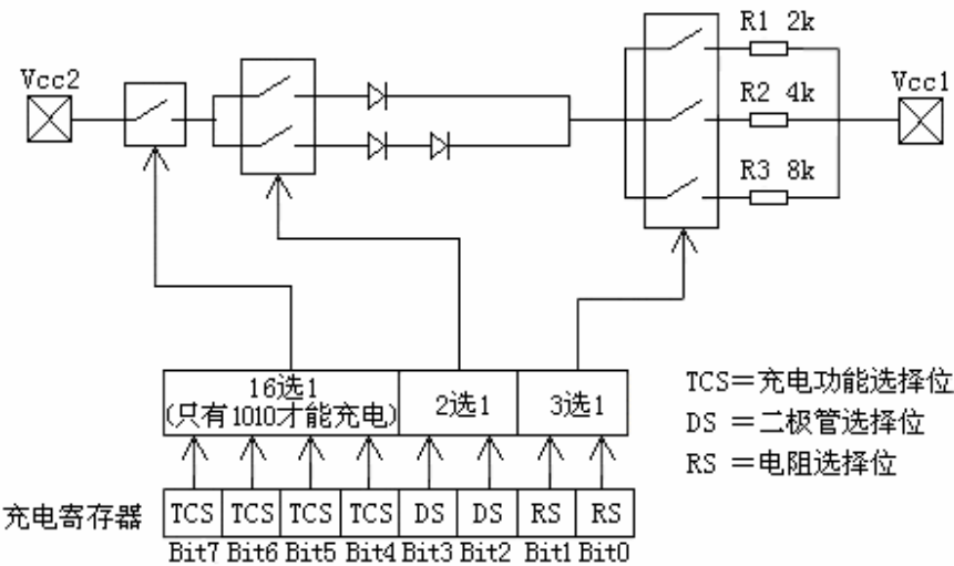
图 4 HYM1302 可编程慢速充电器
