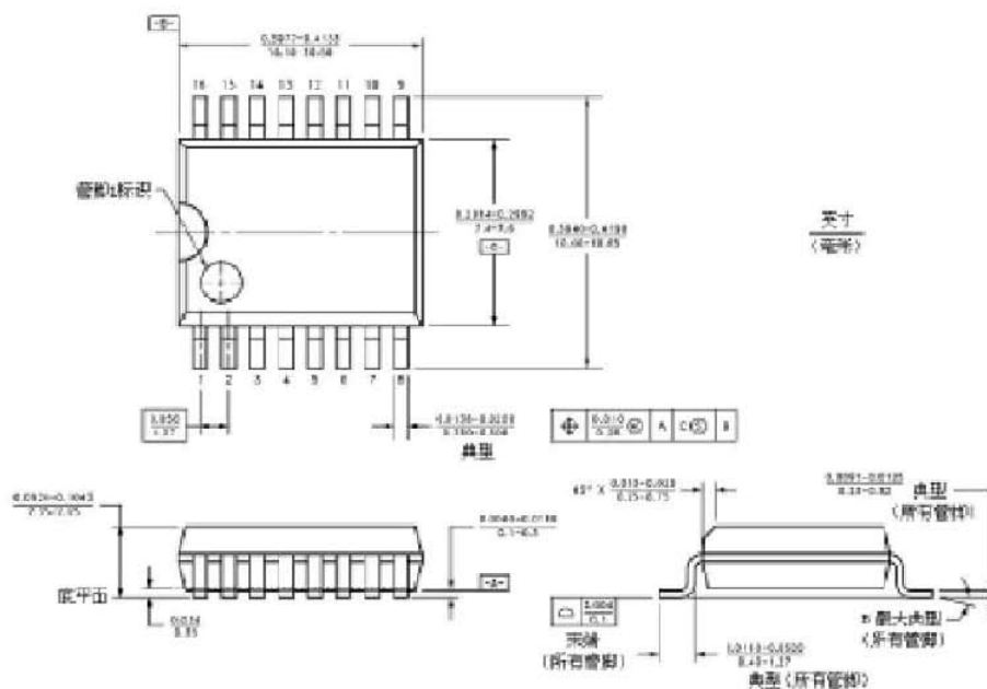
SOP—16/DIP-16 封装结构尺寸图
