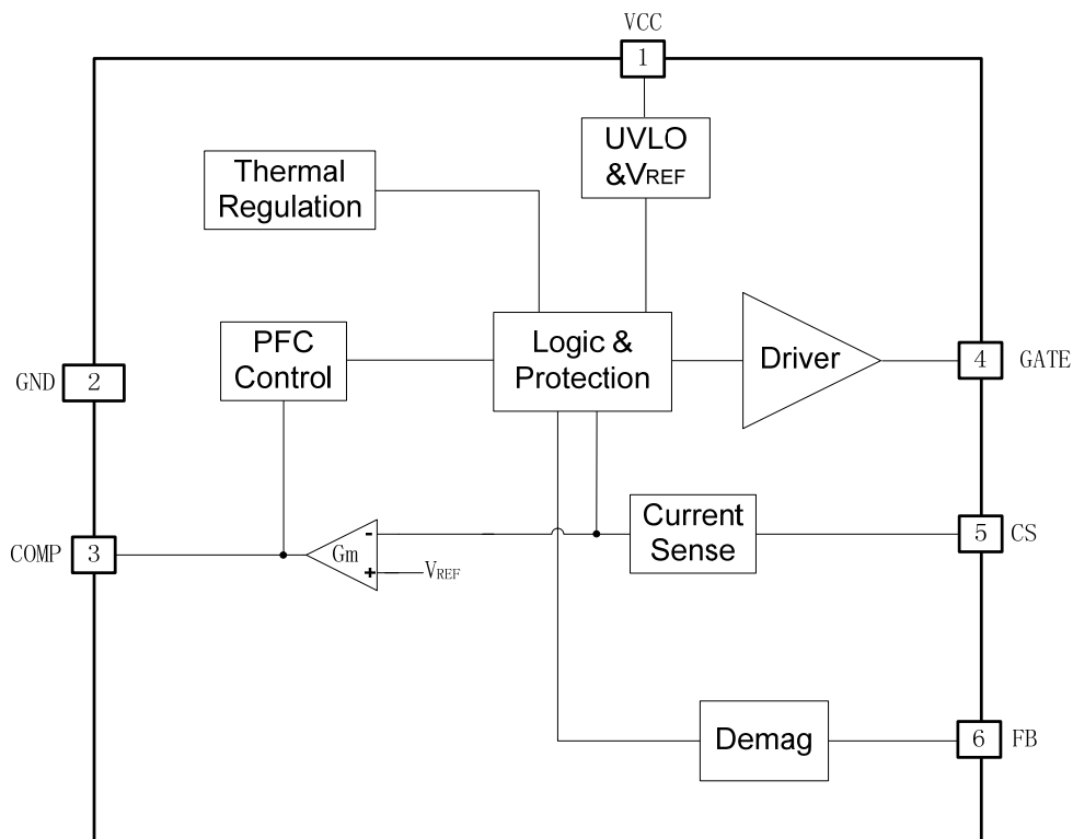
图 3 HW9019B 内部框图
