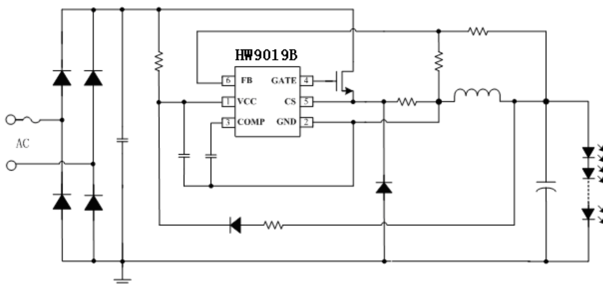
图 1 HW9019B 典型应用图
