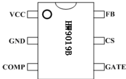
图 2 管脚封装图
