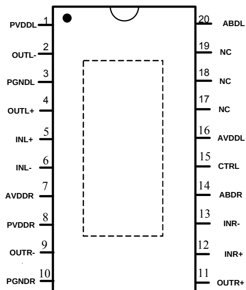
HT8697 顶视图
