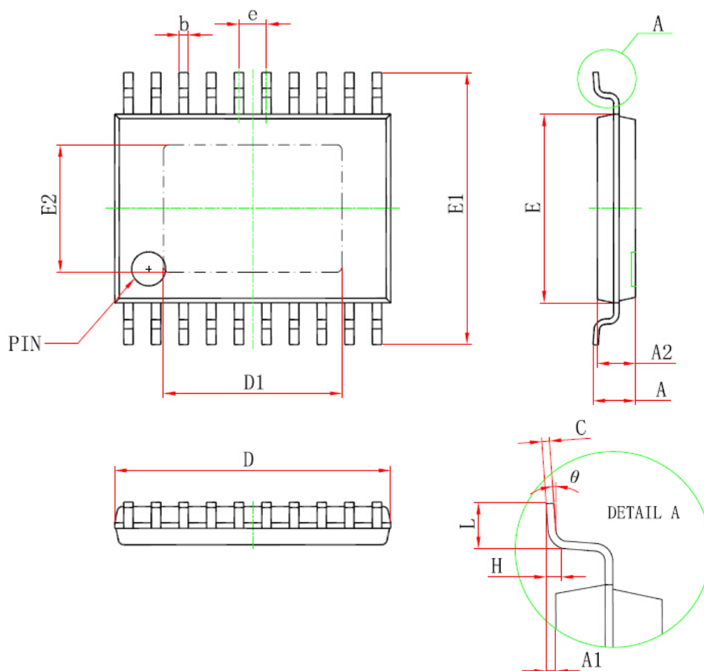
TSSOP20-PP Package
