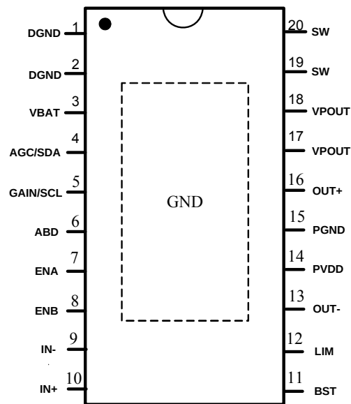
TSSOP20L-PP 顶视图
