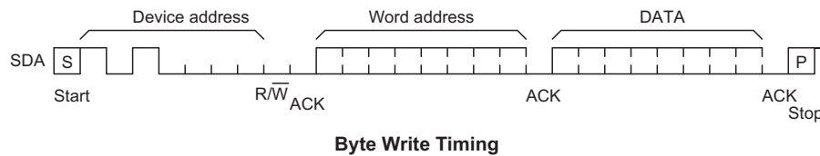
Byte Write Timing
