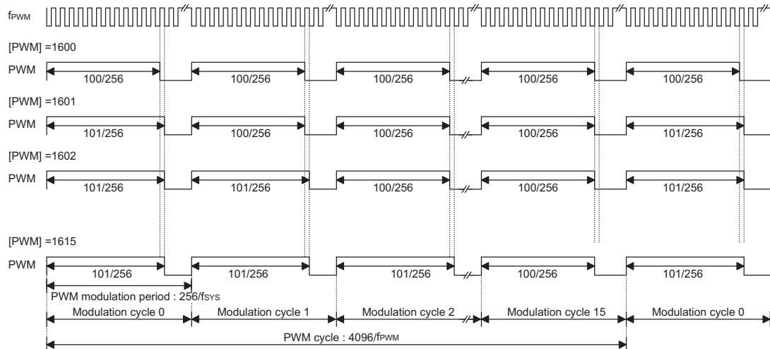
8+4 PWM Mode
