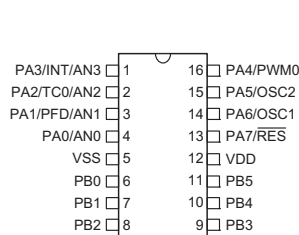
HT46R064 16 DIP-A/NSOP-A
