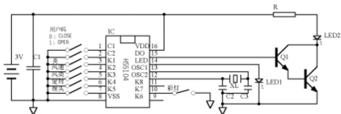
HS5104 发射器线路图
