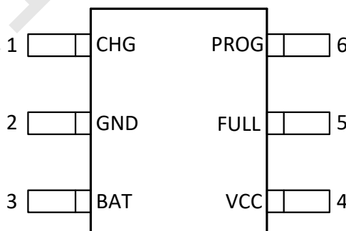
SOT23-6L 顶视图
