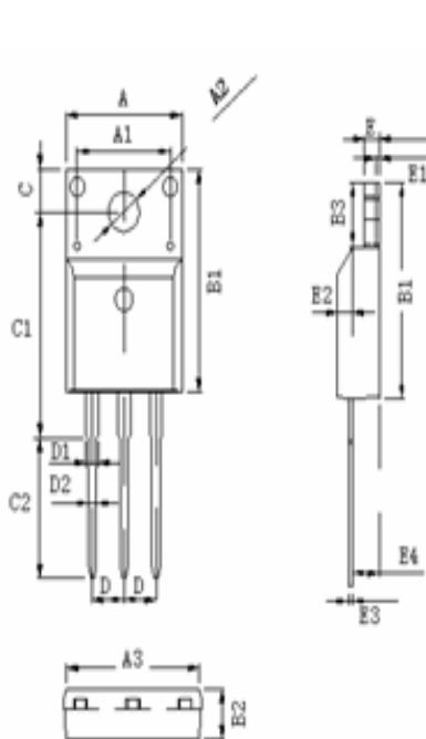
TO-220F 外形尺寸图
