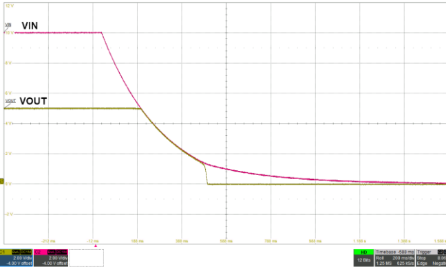
Fig 7. VIN power off
