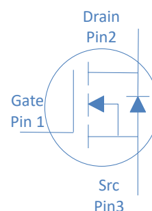
TO-263
