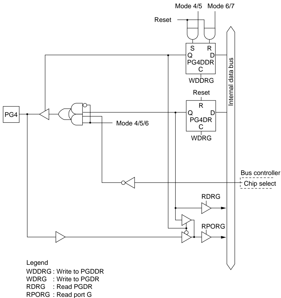
Figure C-15 (d) Port G Block Diagram (Pin PG4)
