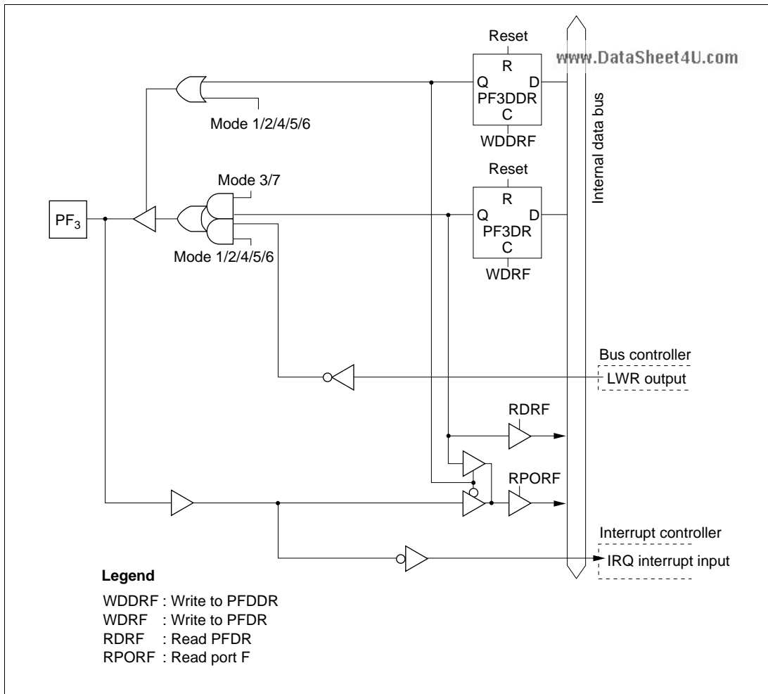
www.DataSheet4U.com Figure C.10 (d) Port F Block Diagram (Pin PF 3 )
