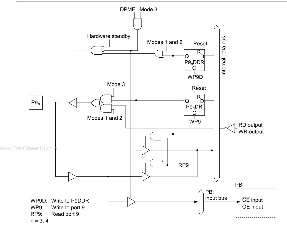
Figure C.9 (d) Port 9 Block Diagram (Pins P9 3 , P9 4 )
