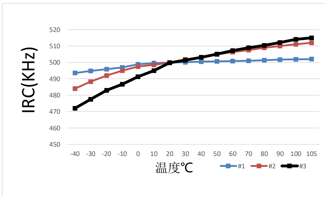
Figure 21-3 内部高频 RC32M/64-温度特性曲线图
