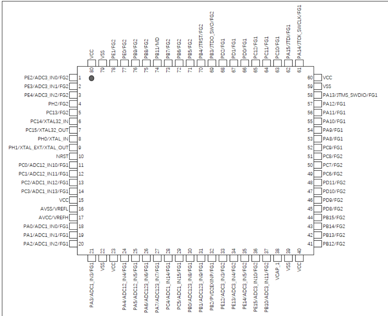
LQFP80
