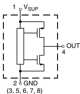
SOIC8 package
