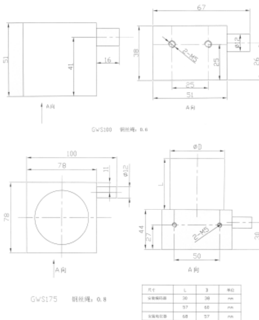
外形尺寸图：
