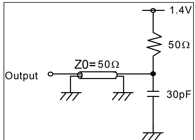
LVTTL A.C. Test Load (B)
