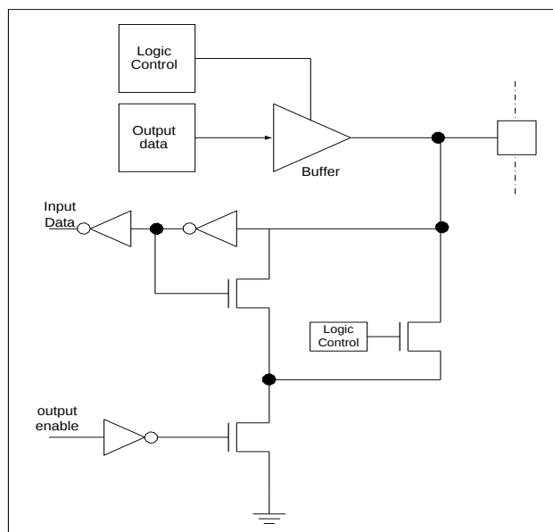
IOAB.0-7: Input/Output Port
