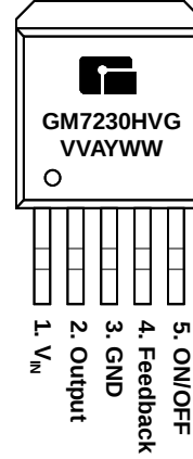
TO-263-5
