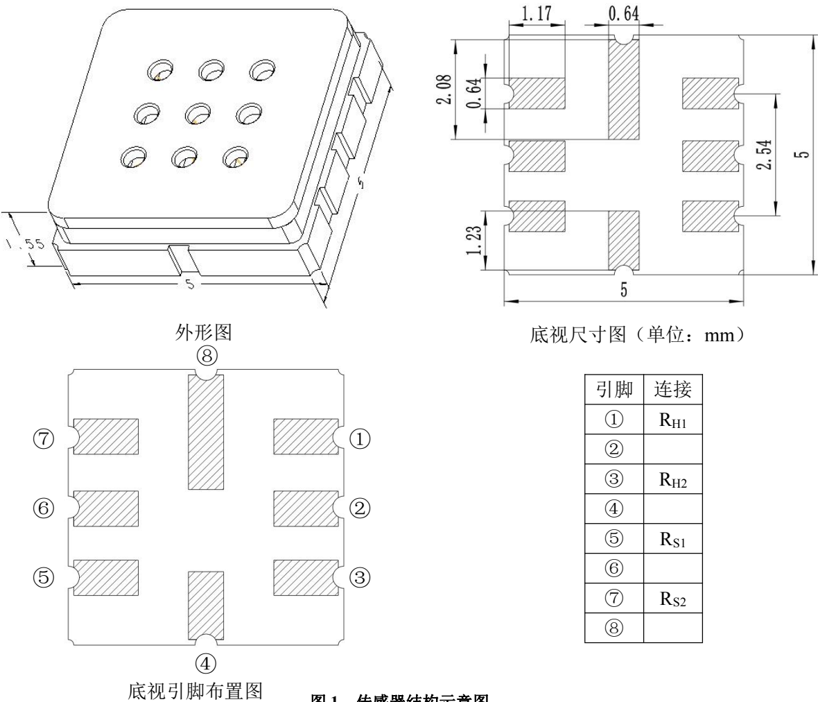
图 1 传感器结构示意图
