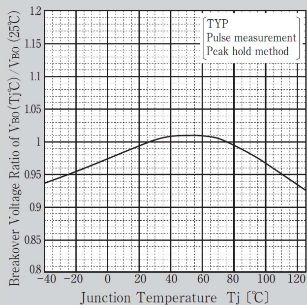
V_{BO} - T_J 特性
