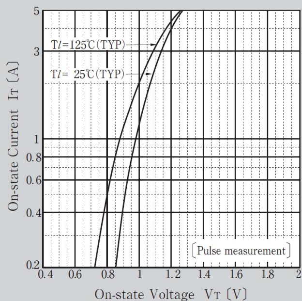
オン電圧 - オン電流
