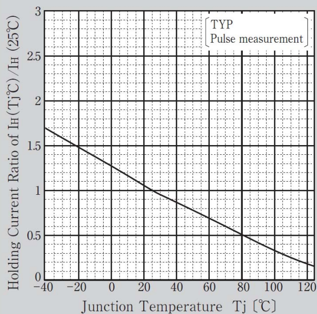
I_H - T_J 特性
