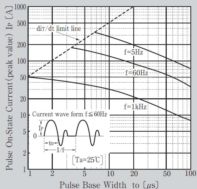
せん頭パルス電流
