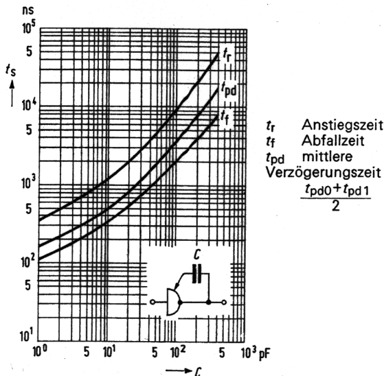
Bild 5 Verlängerung der Schaltzeiten t_s in Abhängigkeit von der Integriertkapazität C bei U_{Batt}=12 V.
