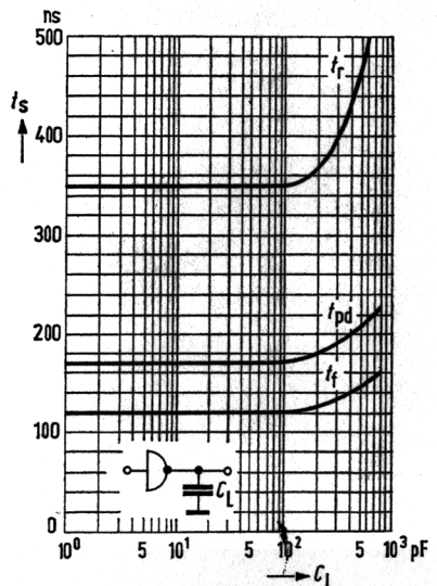
Bild 6 Abhängigkeit der Schaltzeiten t_s von der Lastkapazität C_L bei U_{Batt}=12 V.
