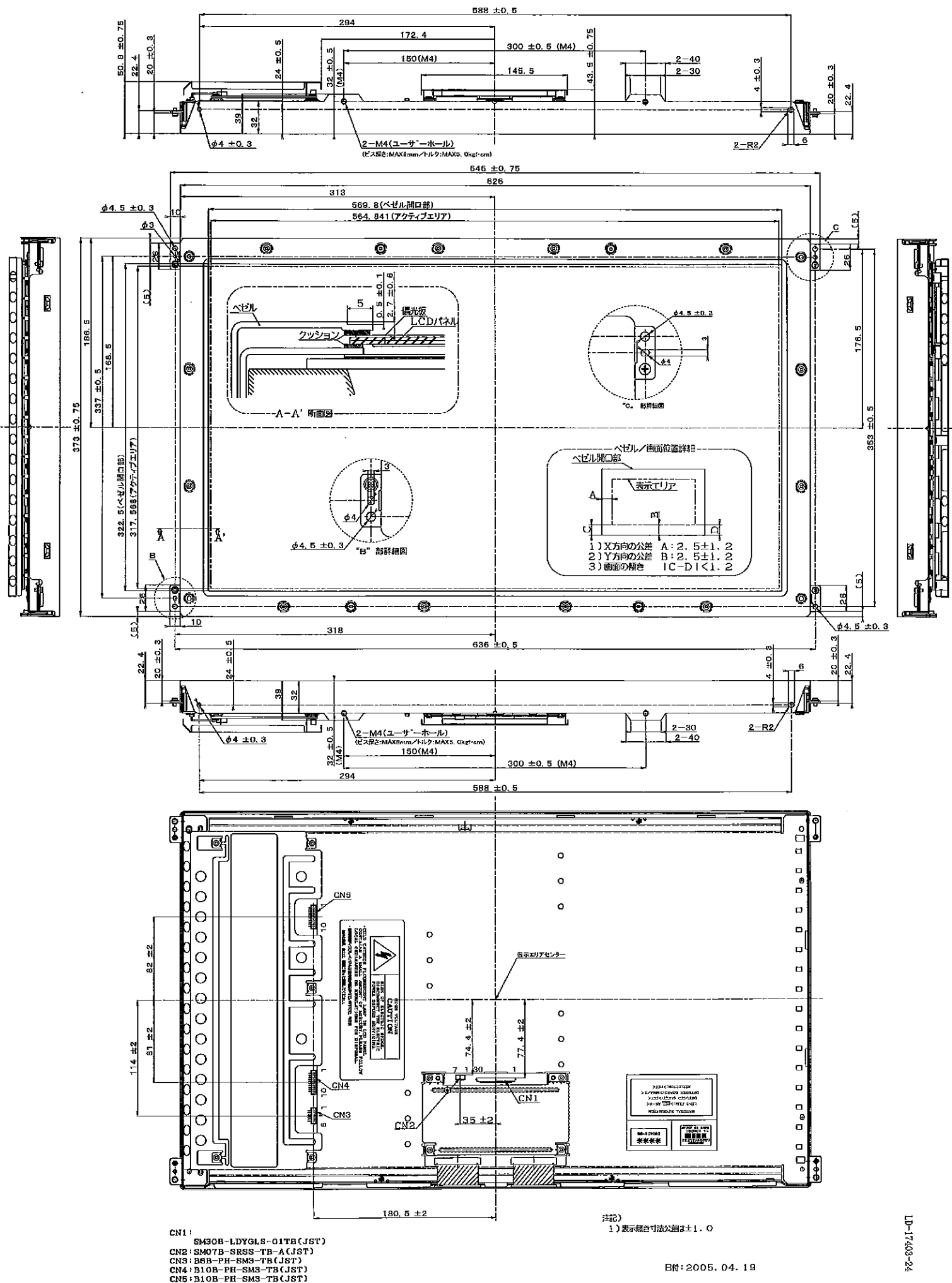
TFT-LCDモジュール外形図
