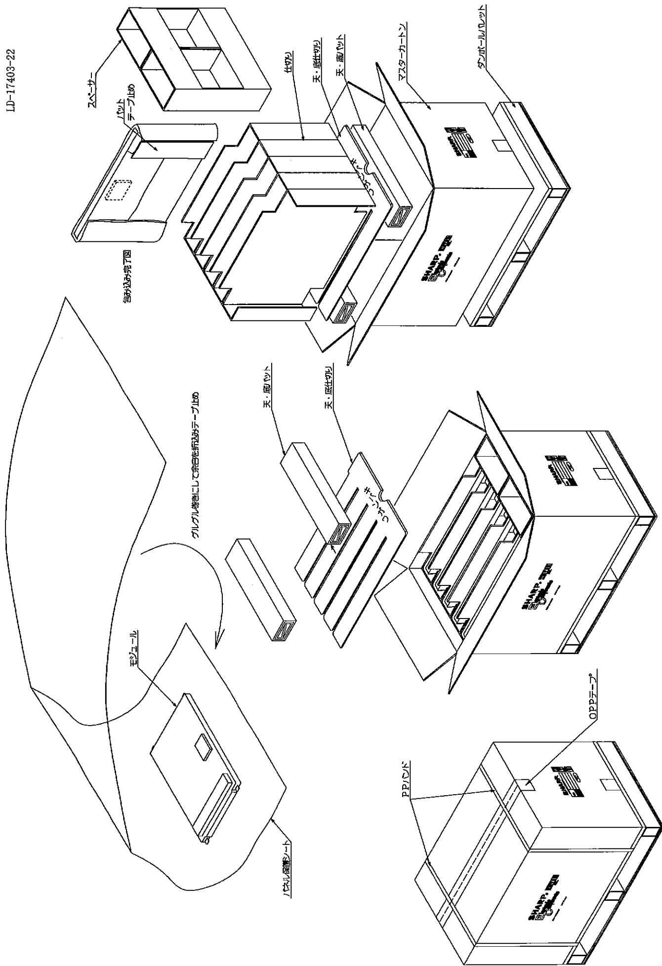
図4-1 LQ255T3LZ24 梱包形態図
