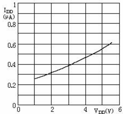
图5. CLKOUT=32.768kHz, I DD 与V DD 的关系图
