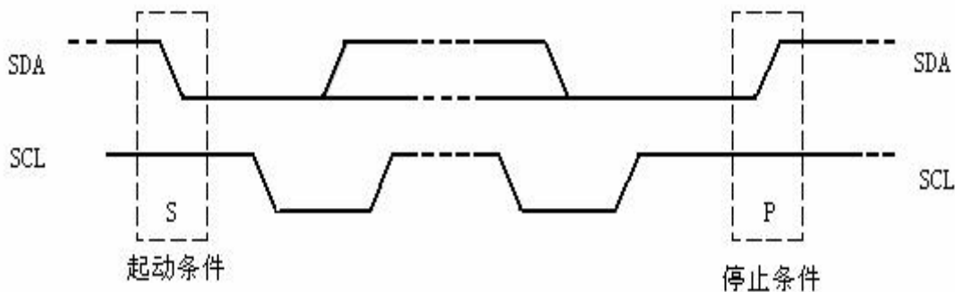
图11: I2C总线的起动 (START) 和停止 (STOP) 条件定义
