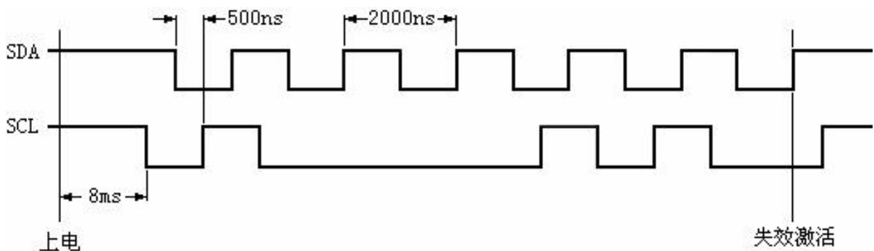
图9. POR失效时序图
