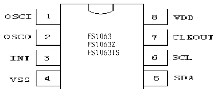
图2. 管脚配置
