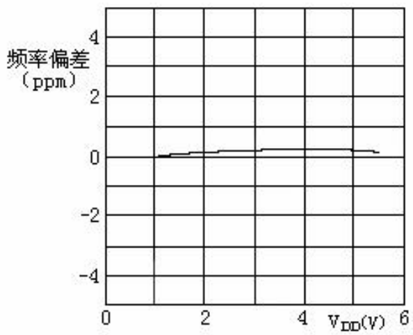
图7. 频率偏差与V DD 的关系图
