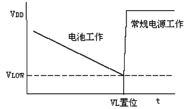
图8 掉电检测
