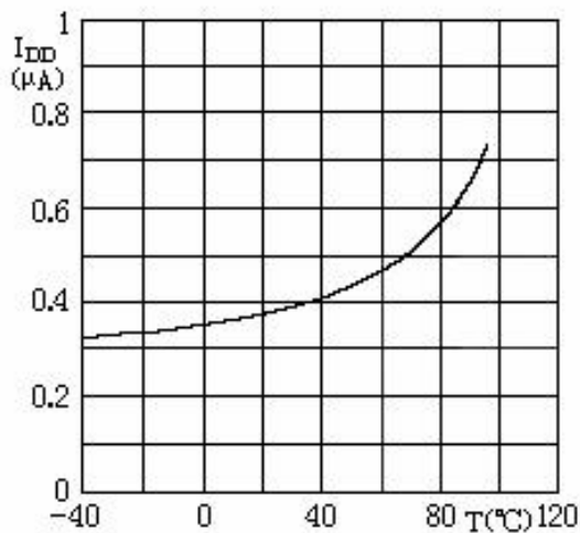
图6. CLKOUT=32.768kHz, I DD 与T A 关系图
