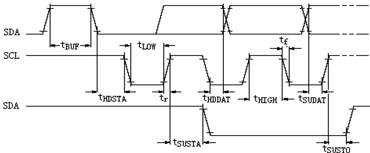
图3 PC总线时序波纹
