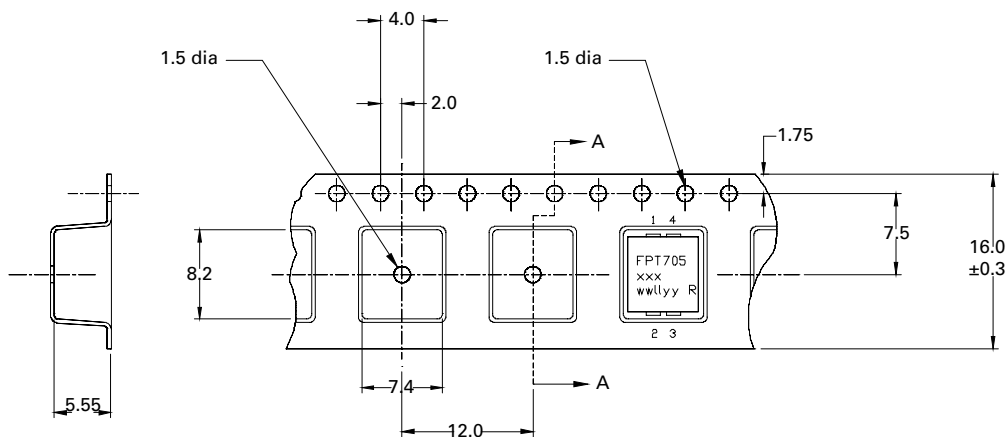
Section A-A
