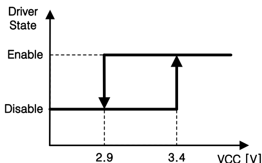
Figure 28. UVLO
