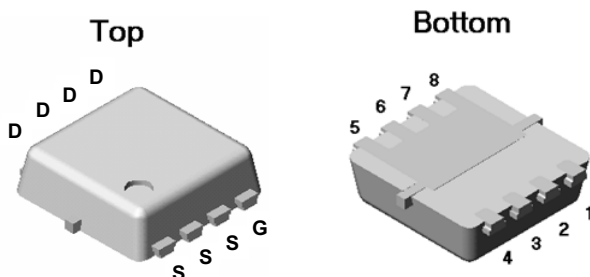
MLP 3.3X3.3
