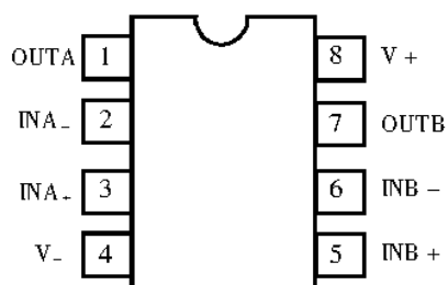
DIP、CSOP 型
