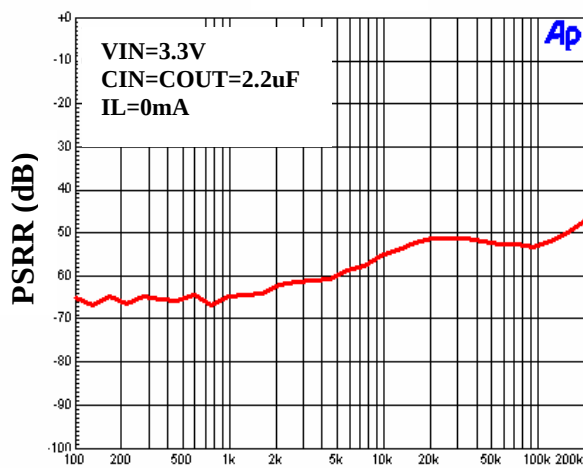
PSRR
