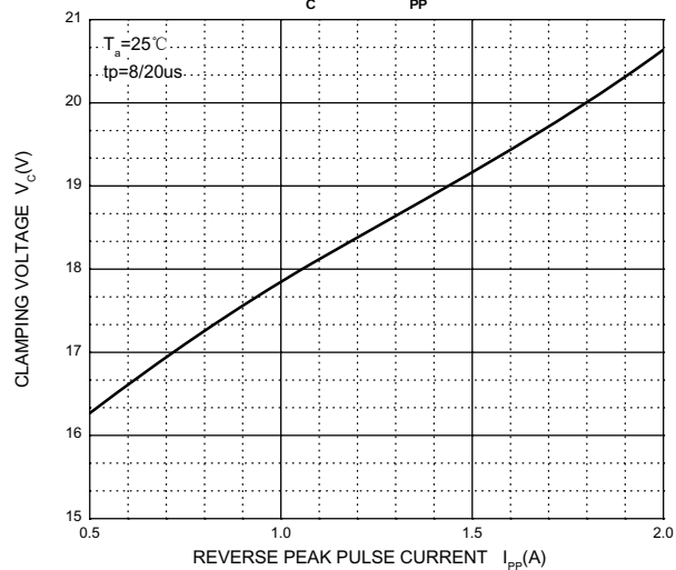
V_C — I_{PP}
