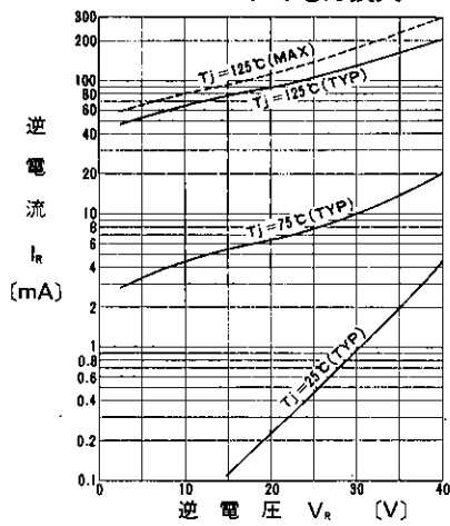
逆特性
