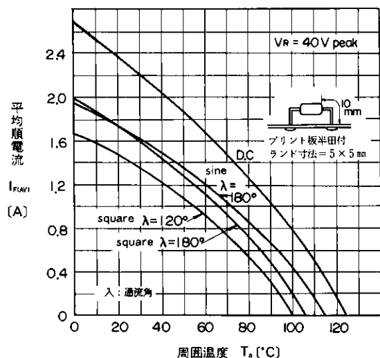
平均順電流—周囲温度特性 I_{F(AV)} - T_a Characteristics
