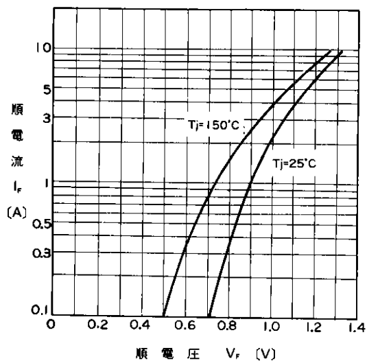
順特性（代表特性） Forward Characteristics
